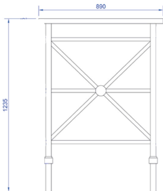
VISTA FRONTALE
