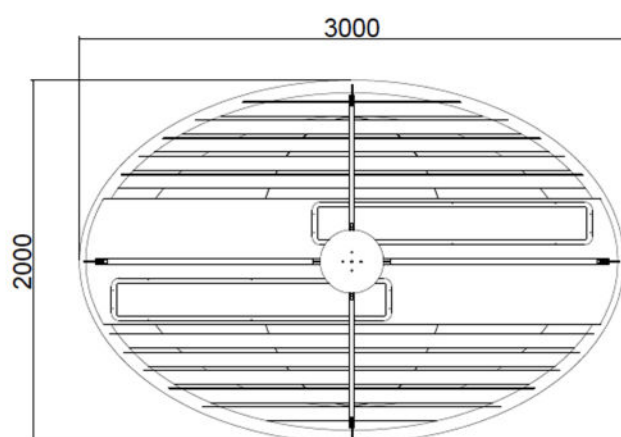
VISTA SUPERIORE
