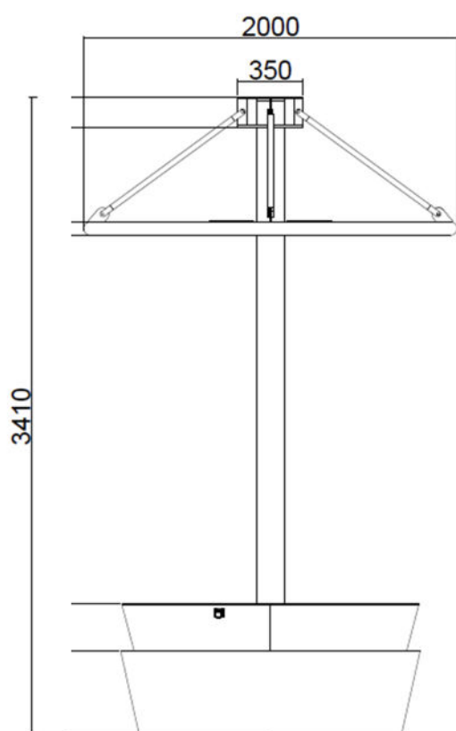
VISTA FRONTALE
