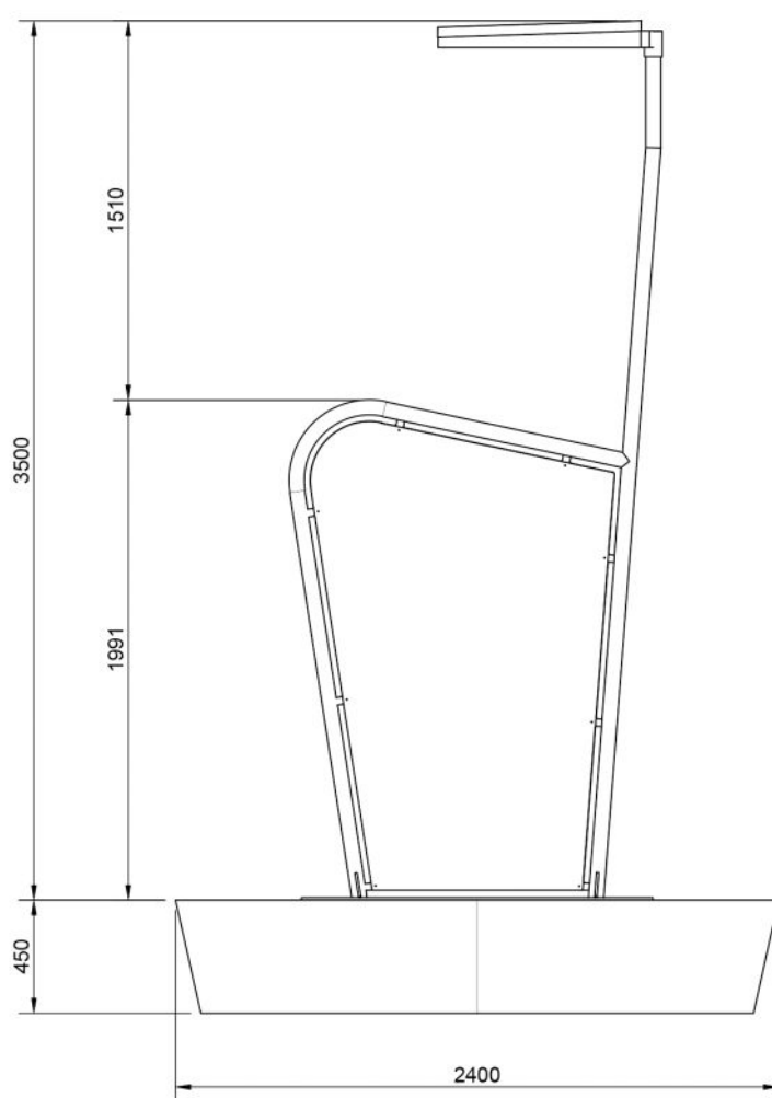
VISTA FRONTALE
